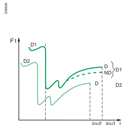
Diagramme énergie.
