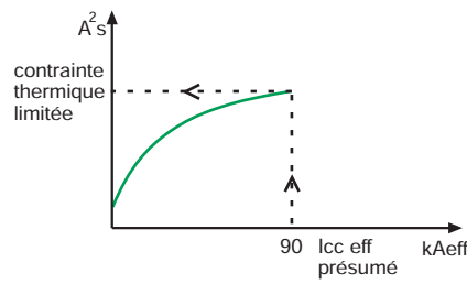
Courbe de limitation en contrainte thermique.
