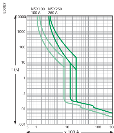
Diagramme temps/courants.
